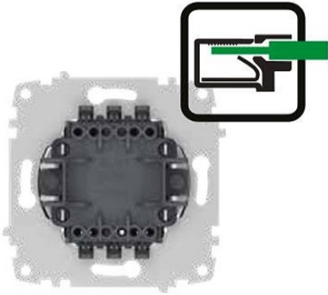
Quick Connect (screwless) Hızlı Bağlantı (vidasız)
