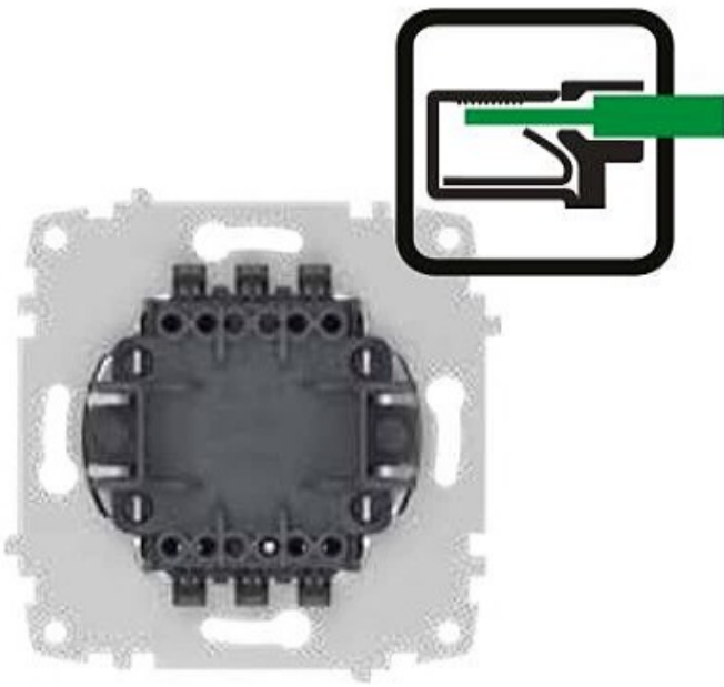
Quick Connect (screwless) Hızlı Bağlantı (vidasız)
