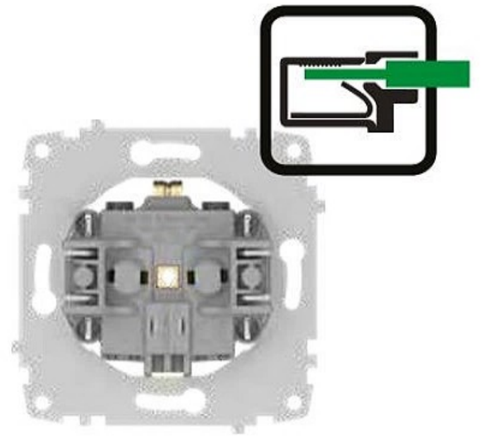
Quick Connect (screwless) Hızlı Bağlantı (vidasız)
