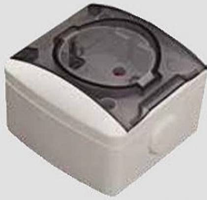
IP54 Child Protection UPS Socket Outlet / IP54 Çocuk Korumalı Kapaklı UPS Priz
